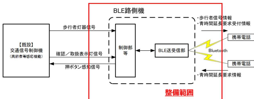
図 2.6-4 UC④のシステム構成
