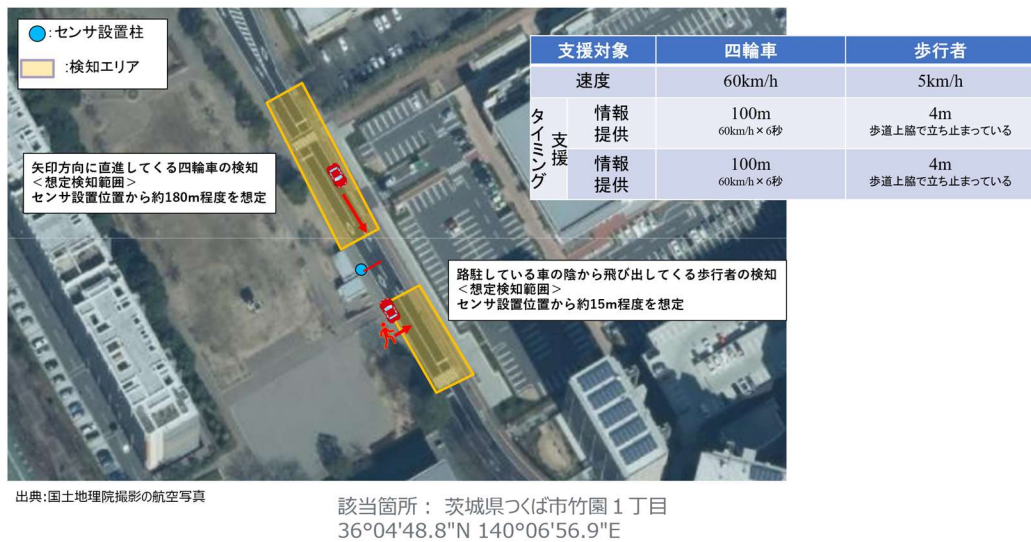
図 2.4-24 UC①-2 センサ設置・検知イメージ②
