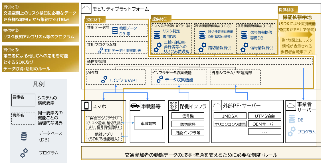
図 2-4 想定システム構成と提供財がカバーする範囲イメージ
